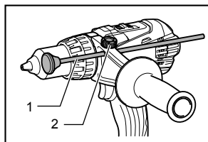
1. Tige de profondeur 2. Vis de serrage
